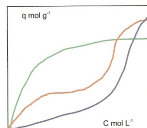
Figura 9.6. Isotermas de adsorción de líquidos.
