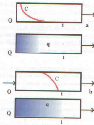
Figura 9.16. Perfil de concentración del contaminante en la fase fluida y captación del contaminante en la fase sólida, al inicio del proceso, b) a un tiempo superior.
